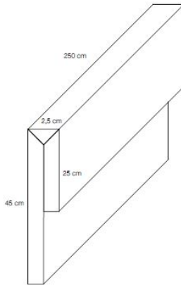
Rohrverkleidung 3- seitig verleimt
